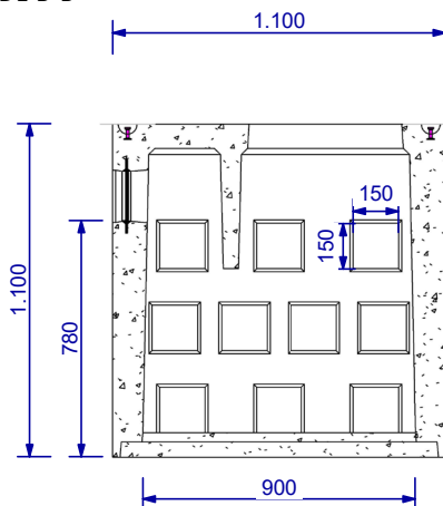
DOORSNEDE B-B
